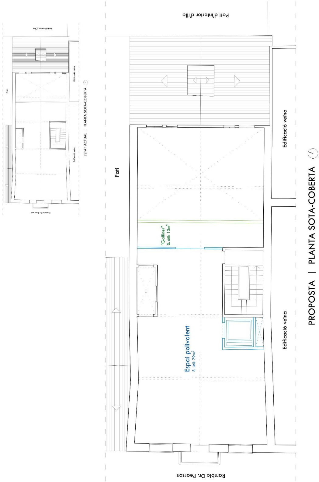
Il·lustració 9: Proposta de distribució de la sota-coberta
